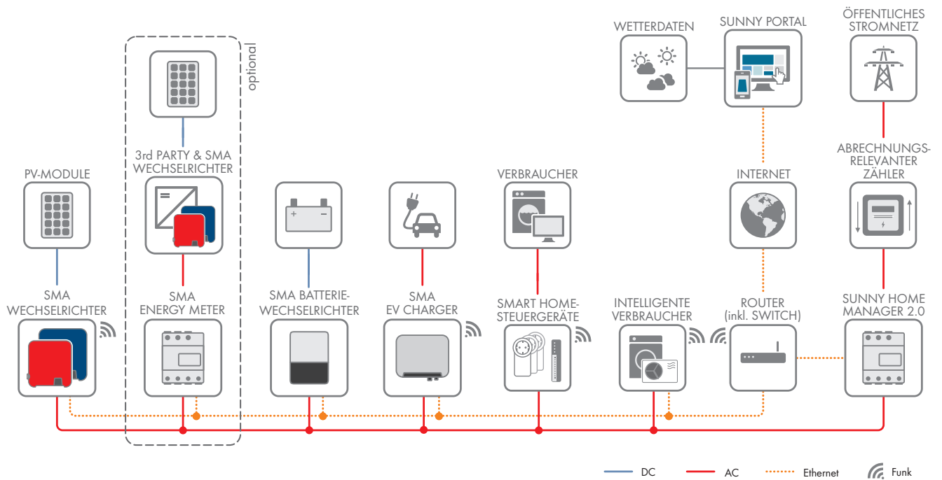
Ilustracja 4: Topologia z systemem magazynowania energii firmy SMA i różnymi sterowanymi odbiornikami (ogólny przykład)
