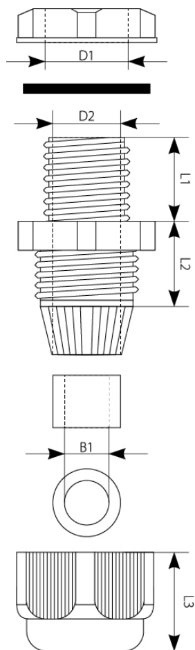
Rysunek Techniczny - Dławnica PG-29, IP68
