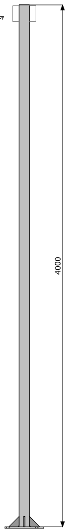
Otwory mocujące maszt fi 25
